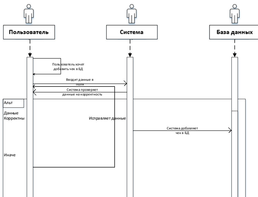
Рисунок 13 - Диаграмма последовательностей прецедента П7 Диаграмма видов деятельности для прецедента П8 «Сформировать отчёт» представлена на рисунке 14.
