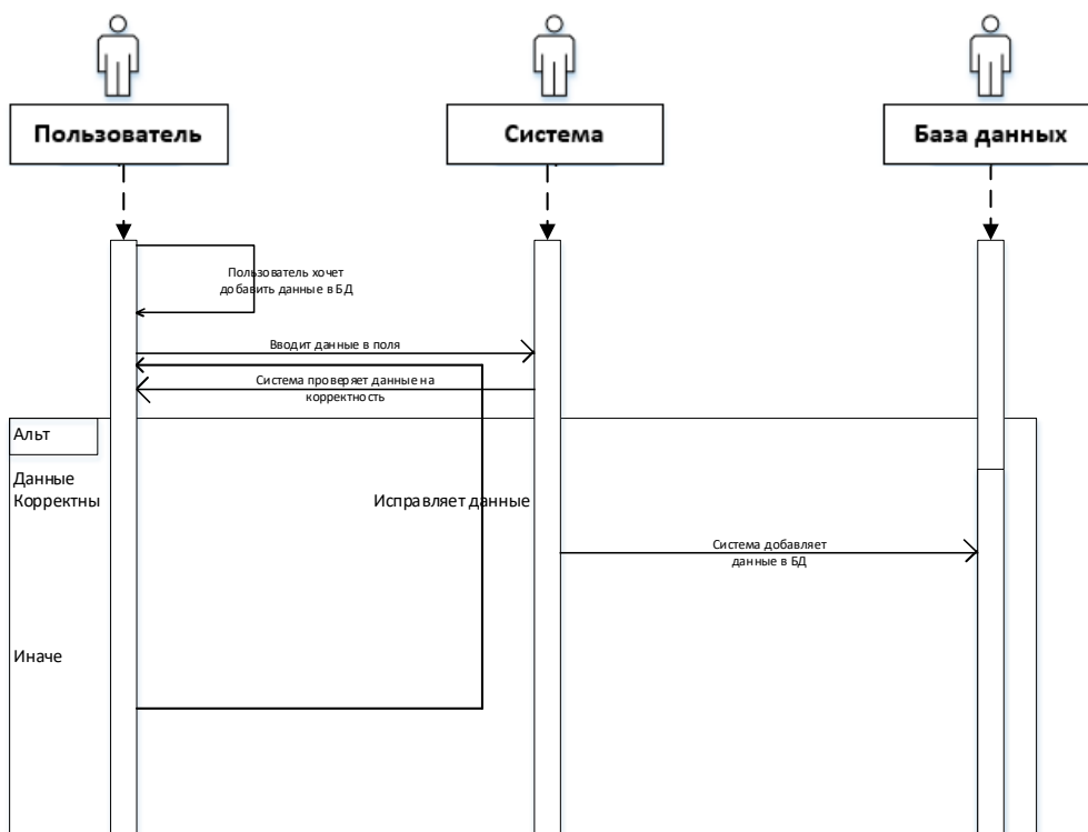
Рисунок 9 - Диаграмма последовательностей прецедента П4 Диаграмма видов деятельности для прецедента П5 «Редактирование записей о товаре» представлена на рисунке 10.
