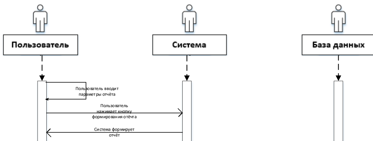
Рисунок 15 - Диаграмма последовательностей прецедента П8 На основании проведенного анализа прикладной системы и спроектированных диаграмм возможно дальнейшая разработка прикладной системы в соответствии с техническим заданием.
