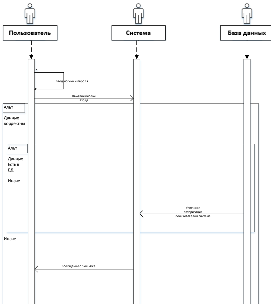
Рисунок 5 - Диаграмма последовательностей прецедента П2 Диаграмма видов деятельности для прецедента П3 «Просмотр данных» представлена на рисунке 6.
