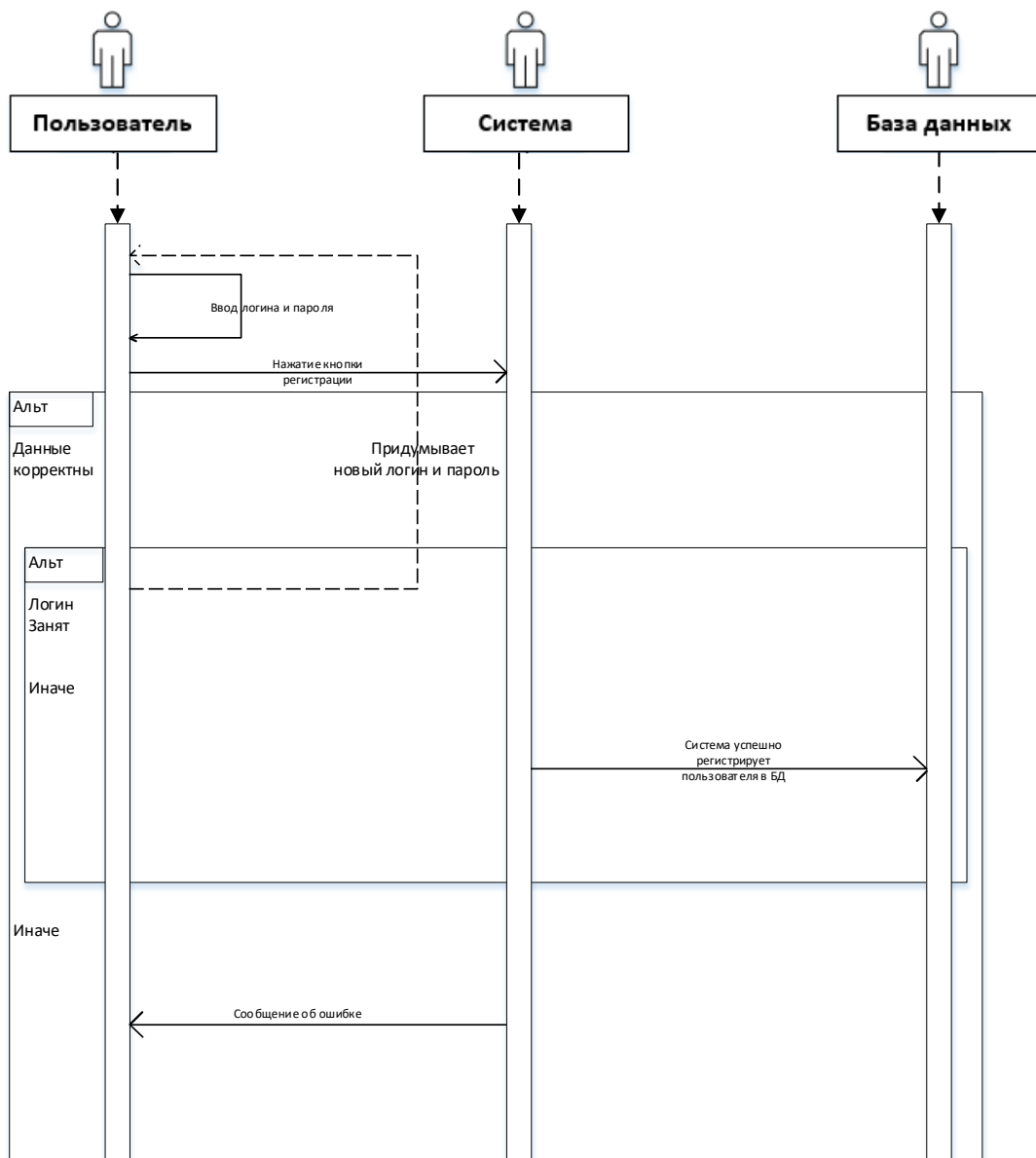
Рисунок 3 - Диаграмма последовательностей прецедента П1 Диаграмма видов деятельности для прецедента П2 «Авторизация» представлена на рисунке 4.
